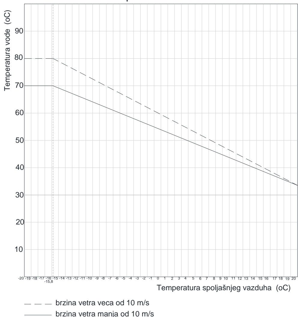
Dijagram promene temperature vode u napojnom vodu toplovodne mreže
